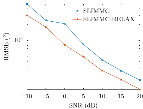
图 5 SLIMMC与SLIMMC-RELAX算法RMSE随SNR变化图 (L=10)
