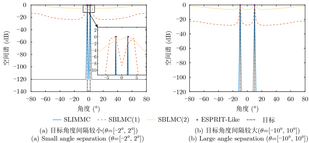
图 9 算法空间谱图( SNR=10 dB)
