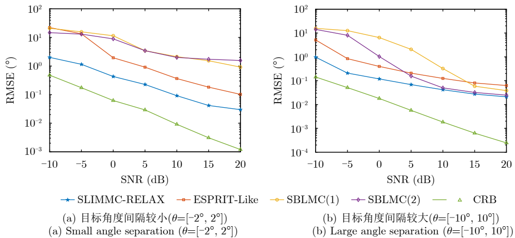
图 10 算法RMSE随SNR变化图
