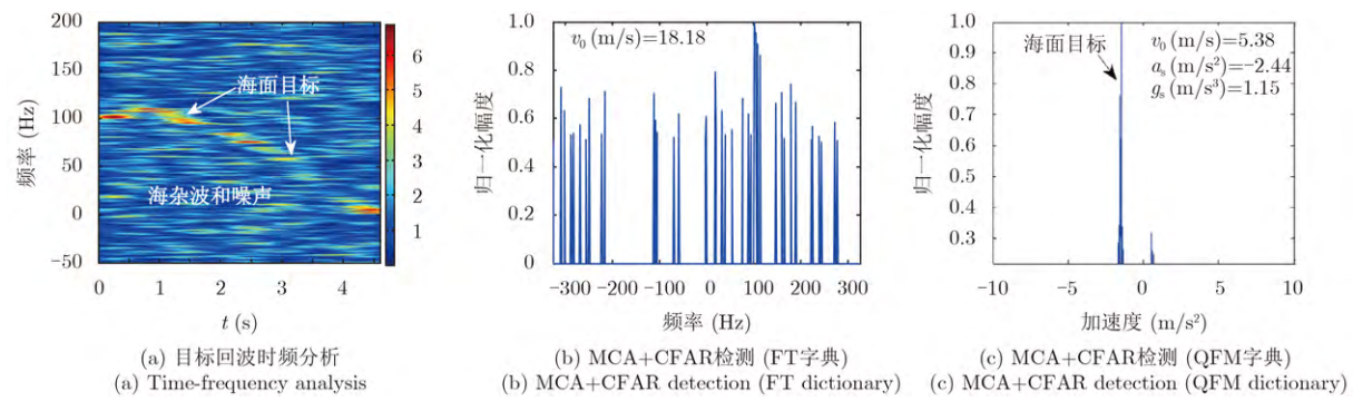
图7 基于MCA海上微动目标检测和特征提取处理结果(S波段雷达数据, P_{fa}=10^{-4} ) [42]
